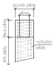
POHLED
