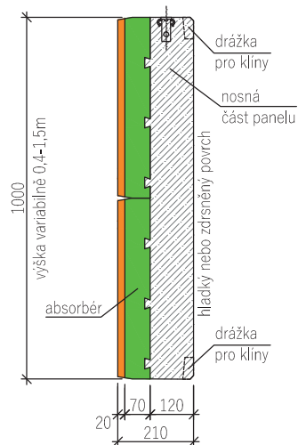
ŘEZ A
