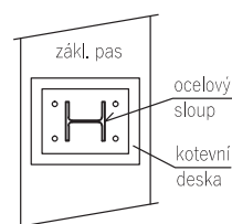
POHLED
