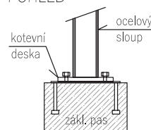
POHLED
