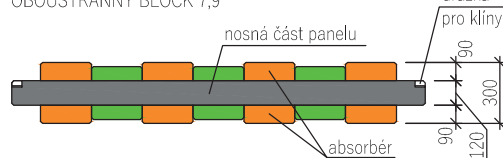
ŘEZ B
