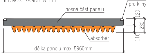
ŘEZ B
