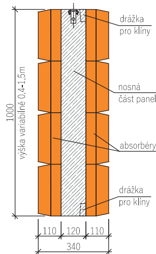
ŘEZ A
