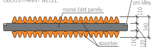
ŘEZ B
